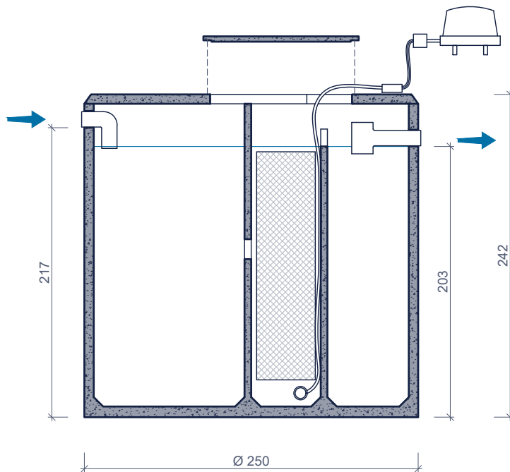
doorsnede coupe
