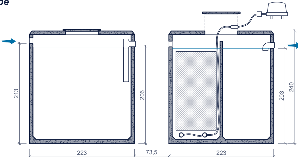
doorsnede coupe
