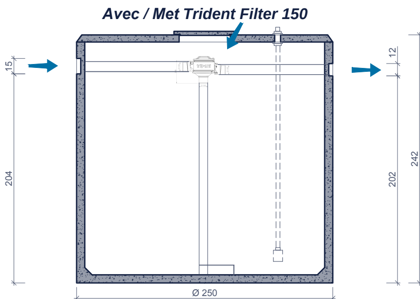
doorsnede coupe
