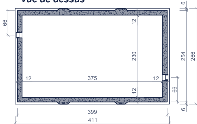
bovenaanzicht vue de dessus
