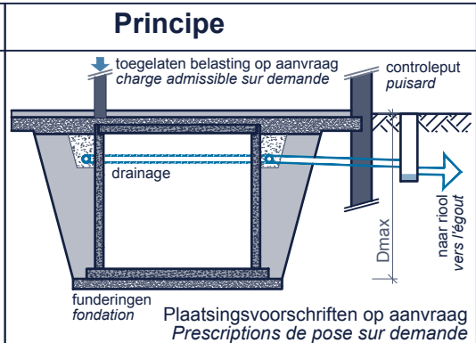
doorsnede met afdekklaar coupe avec couvercle
